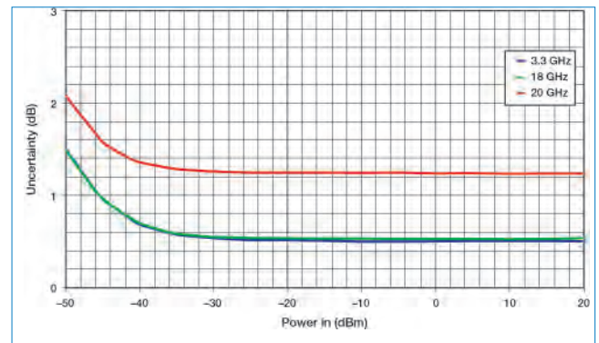
Предполагаемая погрешность монитора мощности при рассогласовании -30 dB для трех частот
